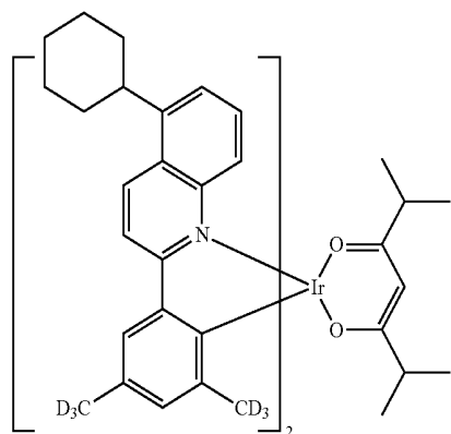
Compound II-43
