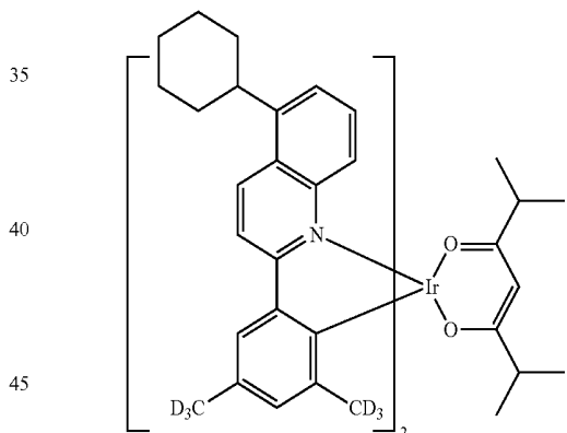
Compound II-43
