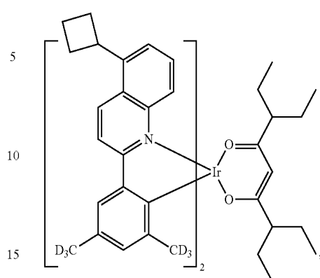
Compound II-49
