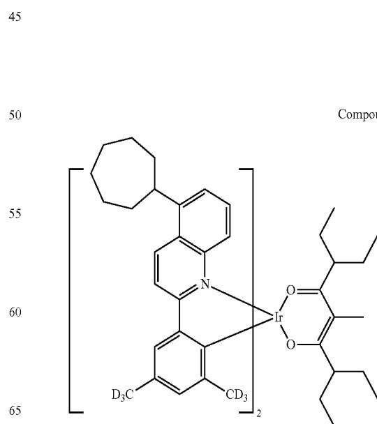
Compound II-49
